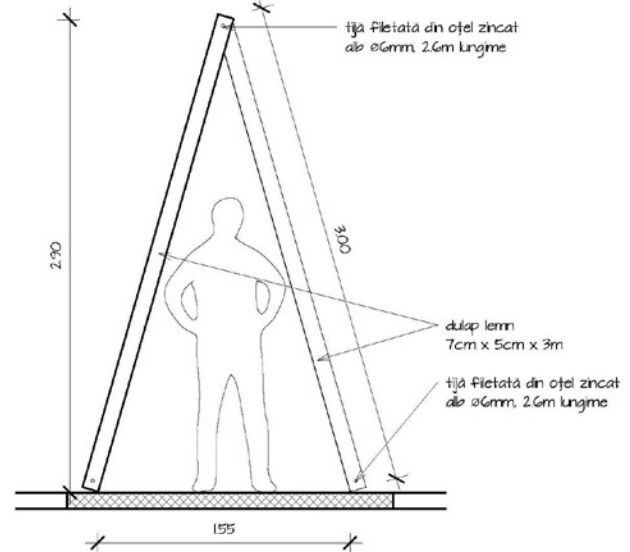
2 Secțiune 1 : 25
