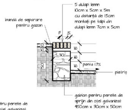
2 Detaliu 3 - Secțiune bancuta 1 : 20
