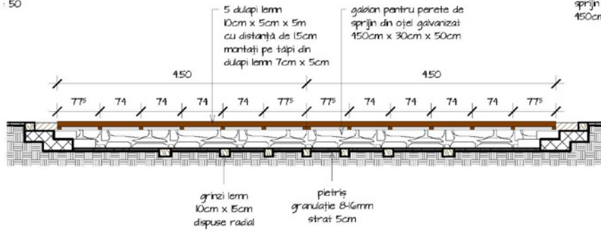
3 Detaliu 3 - Vedere bancuța 1 : 50
