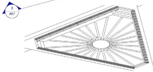
3 Detaliu 3 - Vedere bancuța 1 : 50
